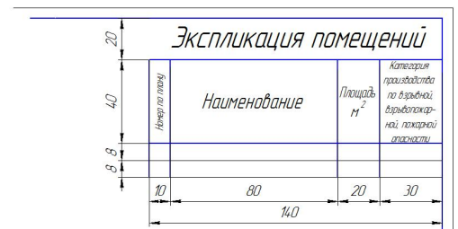
Приложение 2 г) Экспликация помещений производственных корпусов
